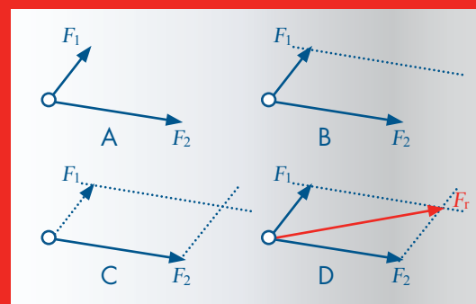
Figuur 4.9: Krachten optellen die in een willekeurige richting staan.
