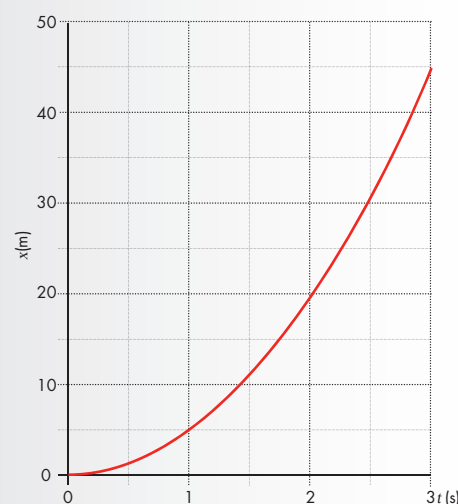
Fig. 2.12: Het (x,t) -diagram bij opgave 12.
