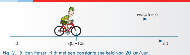
Fig. 2.15: Een fietser rijdt met een constante snelheid van 20 km/uur.
