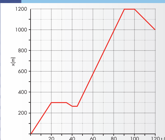
Fig. 2.11: (x,t) -diagram bij opgave 11.
