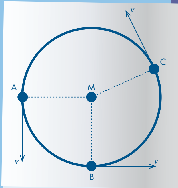
Fig. 3.5: Een cirkelbeweging
