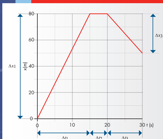
Fig. 2.7: Het (x,t) -diagram van een wandelaar.
