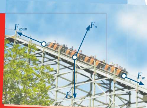
Figuur 4.3: Kracht op het treintje van Robin Hood.
