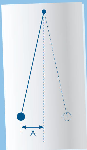
Fig. 3.10: Een slinger
