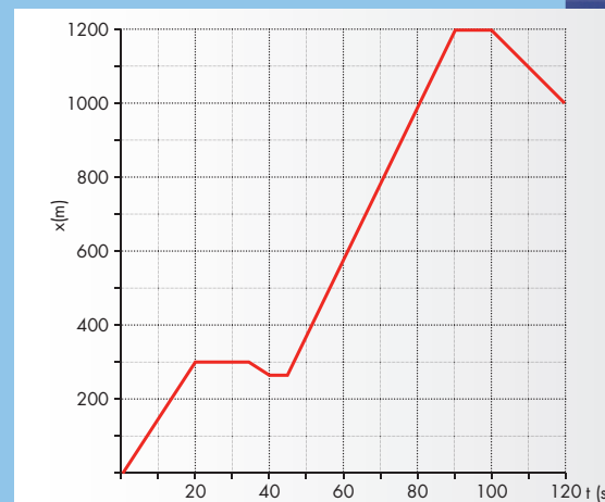
Fig. 2.10: (x,t) -diagram bij opgave 10.
